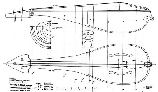
Plans d'un rebec, reconstitué par P. Butler
